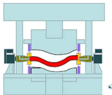
1000tプレス(STAFプロセス)
